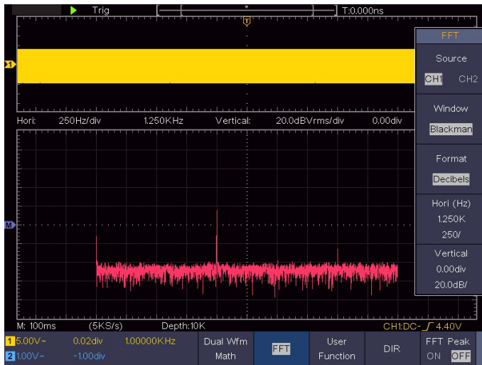
Рисунок 37 - Окно Блэкмена
