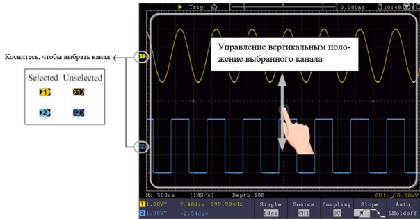
Рисунок 17 - Управление вертикальным положением
