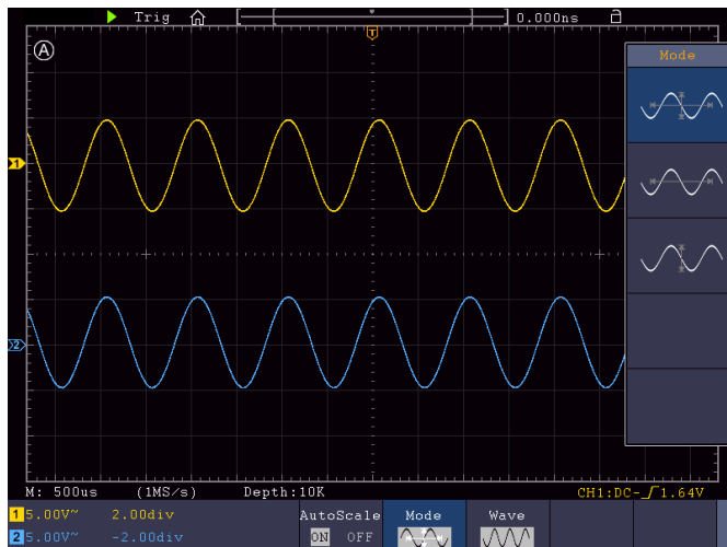
Рисунок 65 - Горизонтально-вертикальное автоматическое масштабирование многопериодных сигналов
