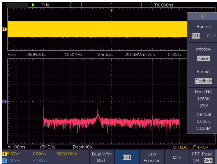
Рисунок 39 - Окно Кайзера
