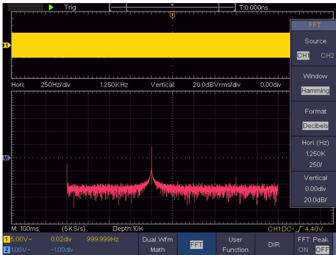
Рисунок 35 - Окно Хэмминга
