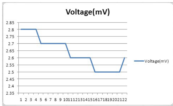
Рисунок 84 - График данных
