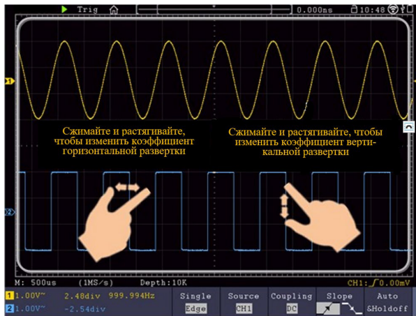
Рисунок 21 - Изменение коэффициента
