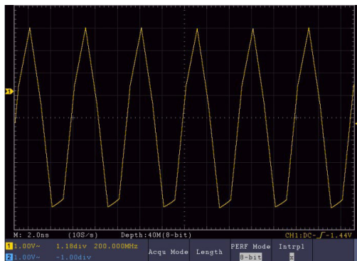
Рисунок 48 - Линейная интерполяция
