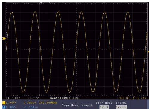
Рисунок 47 - Интерполяция \sin(x)/x
