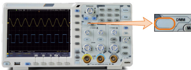
Рисунок 78 - Кнопка мультиметра
