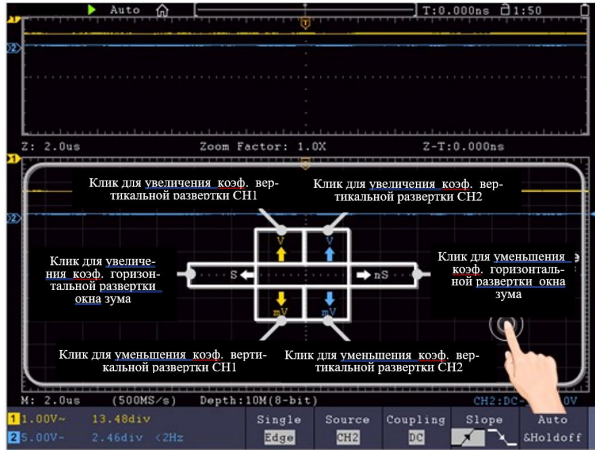
Рисунок 28 - Один зум
