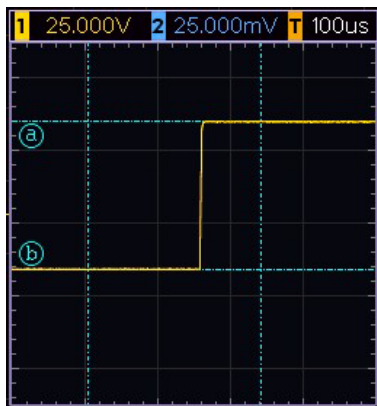
Рисунок 32 - Курсорные измерения
