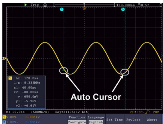
Рисунок 64 - Автоматический курсор
