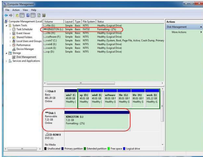
Рисунок 55 - Форматирование USB-диска
