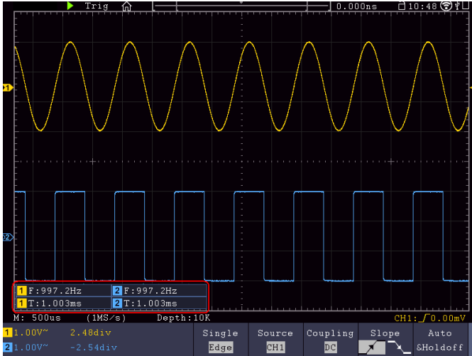
Рисунок 60 - Автоматическое измерение
