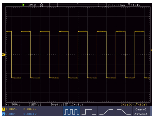
Рисунок 8 - Автоматическая настройка
