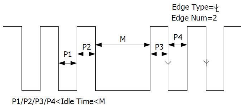
Рисунок 44 - Запуск по N-му фронту
