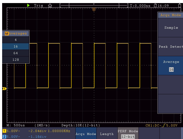
Рисунок 96 - Снижение уровня шума с помощью функции усреднения
