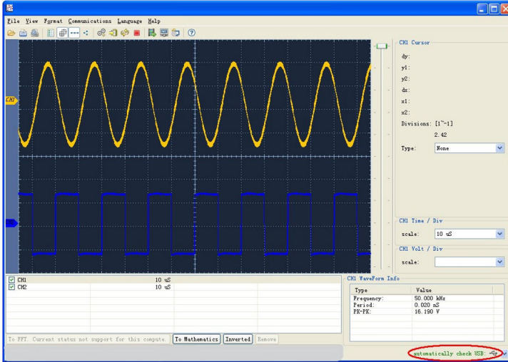
Рисунок 85 - Подключение к ПК через USB-порт
