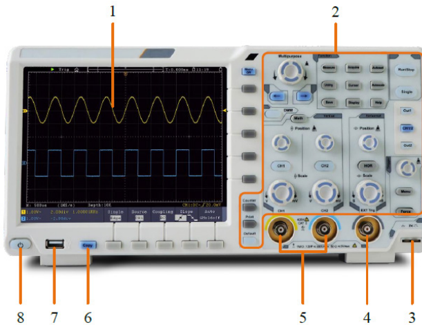
Рисунок 3 - Передняя панель
