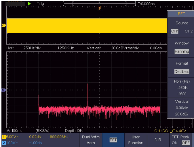
Рисунок 38 - Окно Ханнинга
