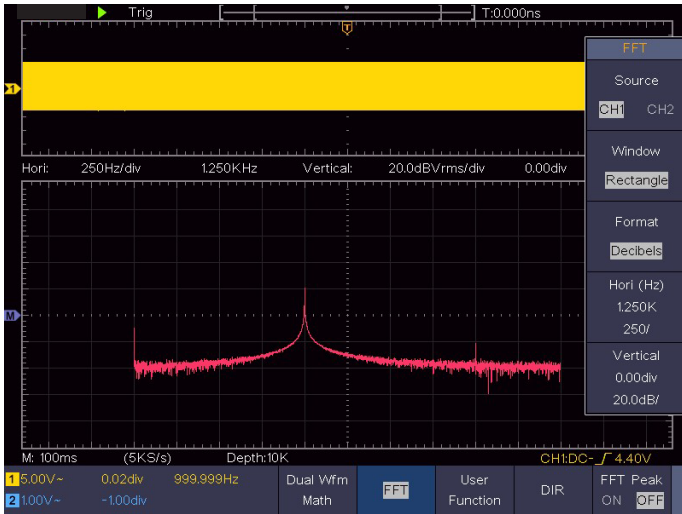
Рисунок 36 - Прямоугольное окно
