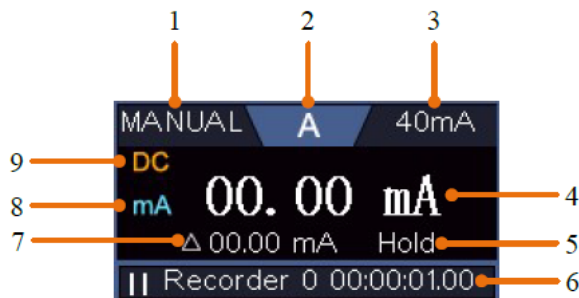
Рисунок 79 - Информационное окно мультиметра
