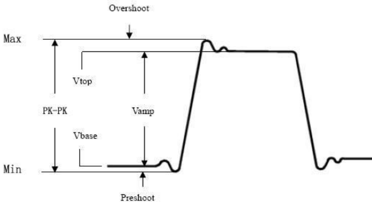
Рисунок 61 - Импульс с некоторыми точками измерения напряжения
