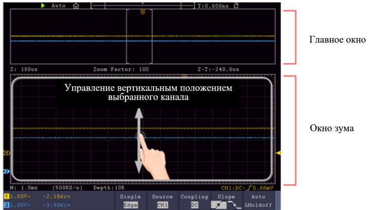
Рисунок 24 - Управление вертикальным положением выбранного канала
