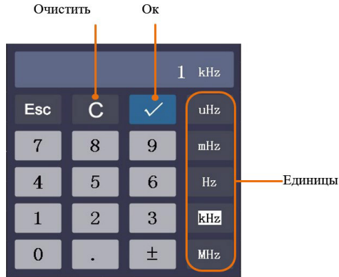
Рисунок 72 - Клавиатура ввода
