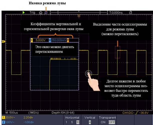
Рисунок 31 - Окно лупы
