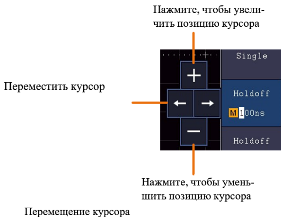
Рисунок 30 - Изменение значений
