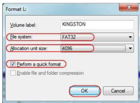
Рисунок 54 - Форматирование USB-диска.
