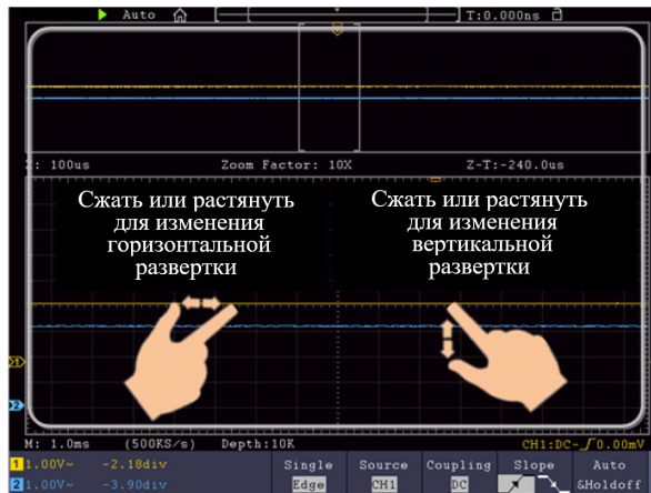
Рисунок 27 - Двойной зум
