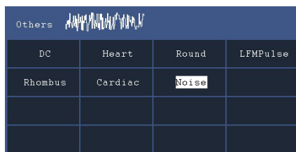
Рисунок 76 - Интерфейс
