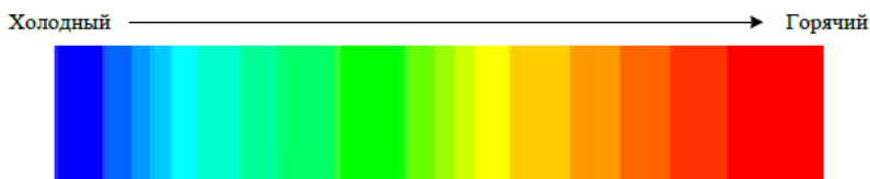
Рисунок 49 - Цветовая градация
