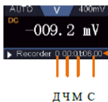
Рисунок 80 - Запись времени
