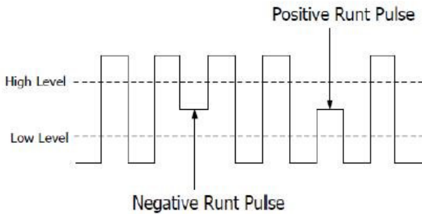
Рисунок 43 - Запуск по ранту (Rant Trigger)
