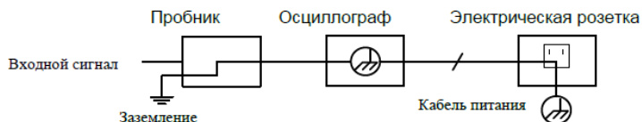
Рисунок 1 - Схема подключения заземляющего провода осциллографа
