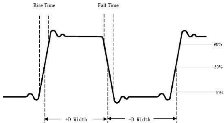
Рисунок 62 - Импульс с некоторыми точками измерения времени
